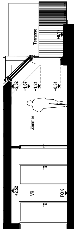
Schnitt
