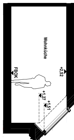
Schnitt
