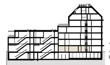
Schnitt
