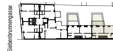
Grundriss 1. Obergeschoss
