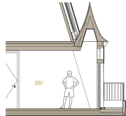
SCHNITT TOP22
