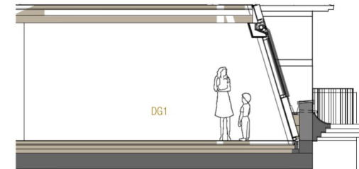
SCHNITT 21
