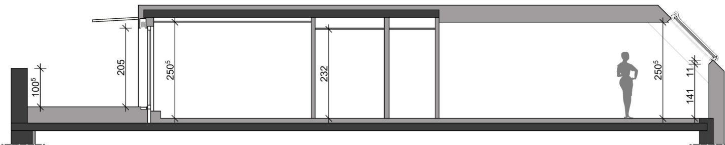
SCHNITT 1-1
