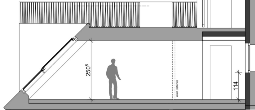
SCHNITT 3-3
