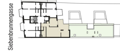
Grundriss 3. Obergeschoss
