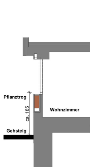
Fassadenschnitt
