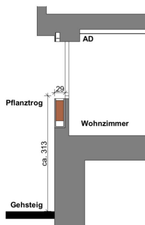
Fassadenschnitt
