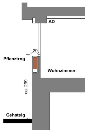
Fassadenschnitt
