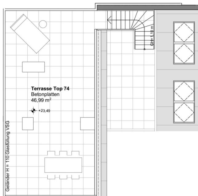
Grundriss Dachterrasse
