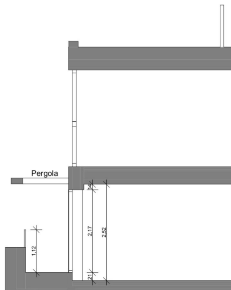
Schnitt 1/74 A
