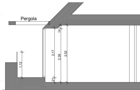
Schnitt 1/75 A
