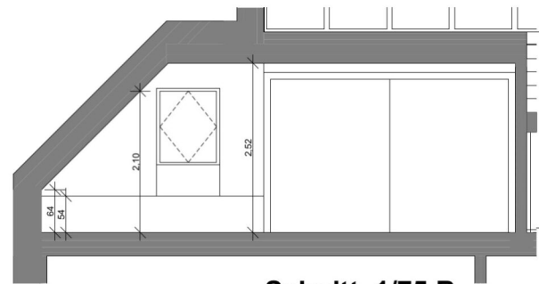
Schnitt 1/75 B
