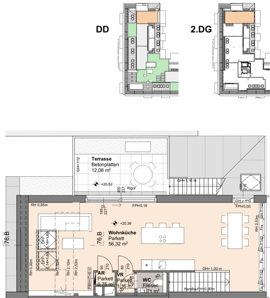
Grundriss 2.Dachgeschoss
