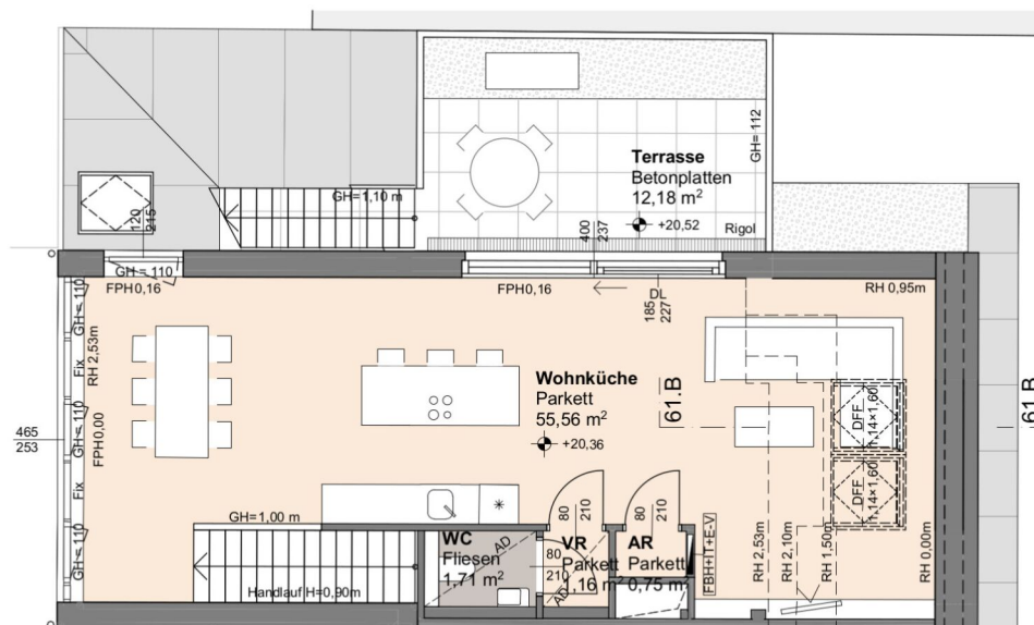
Grundriss 2.Dachgeschoss
