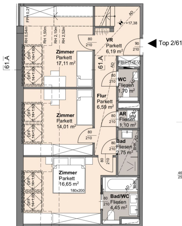
Grundriss 1.Dachgeschoss
