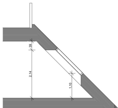
Schnitt 2/61 B
