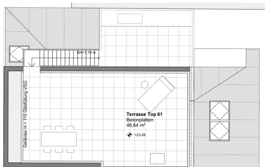
Grundriss Dachterrasse
