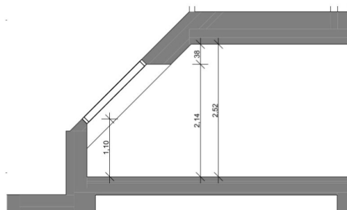
Schnitt 2/61 A
