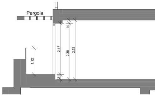
Schnitt 2/67 A
