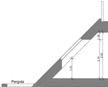
Schnitt 1/79 A
