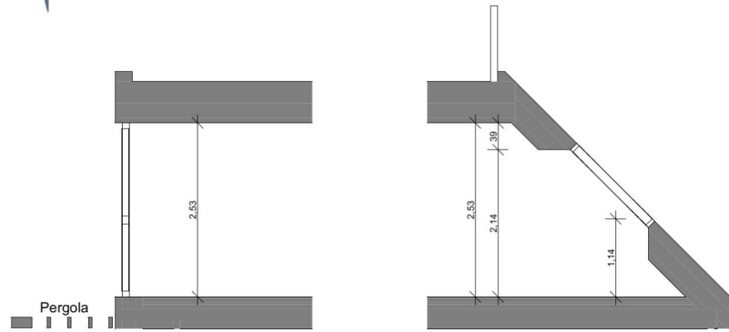
Schnitt 2/70 A
