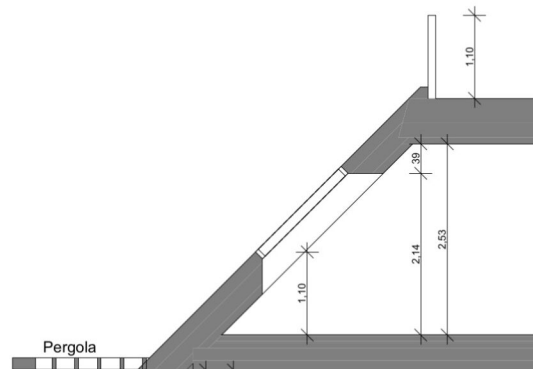
Schnitt 2/71 A
