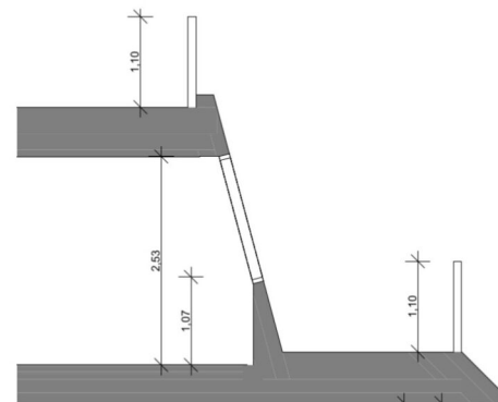
Schnitt 2/71 B
