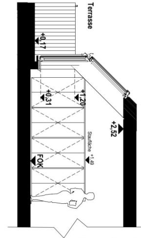
Schnitt 2
