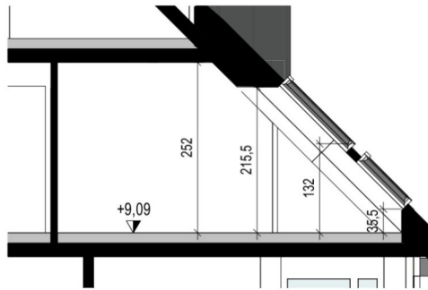
Schnitt 18.A
