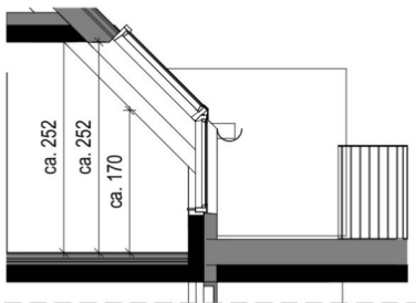
Schnitt 40.A
