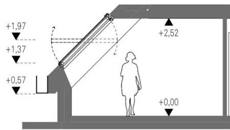
Schnitt 1
