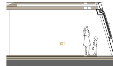
SCHNITT TOP25
