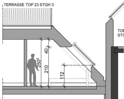
SCHNITT 2-2
