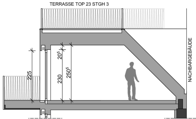
SCHNITT 1-1
