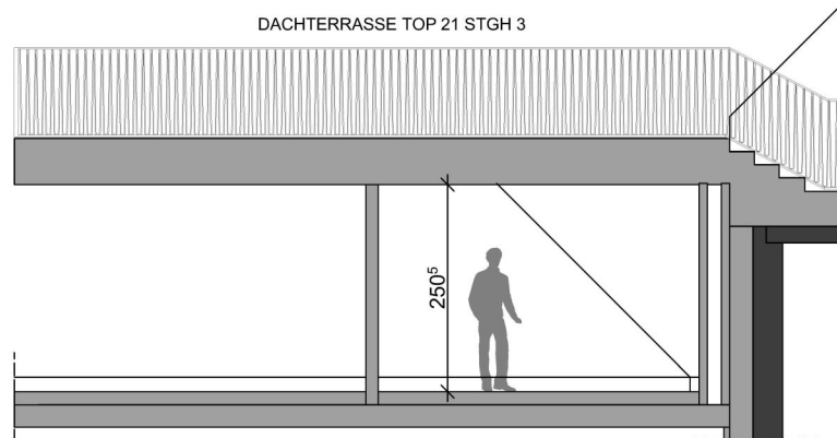
SCHNITT 3-3
