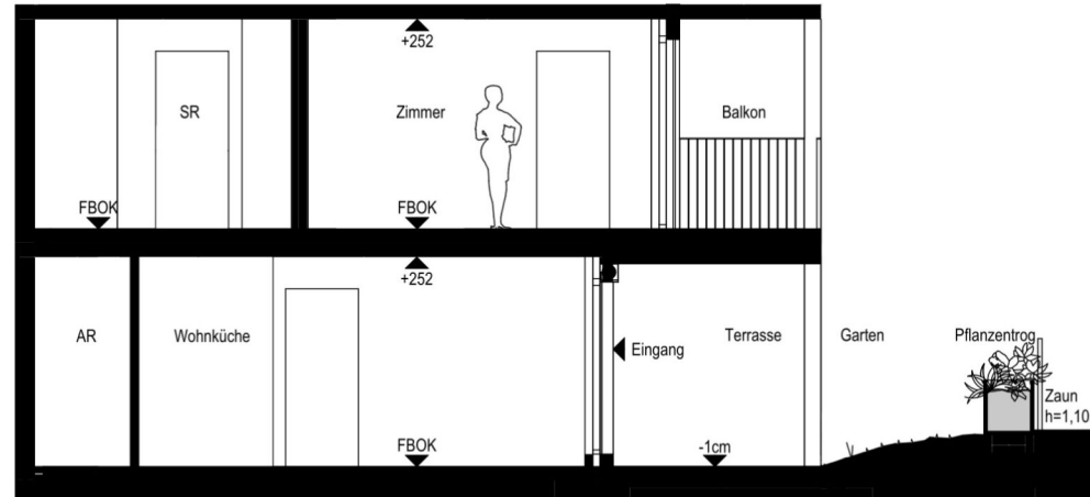
Schnitt S
