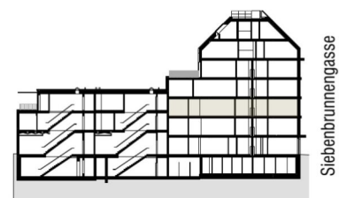
Schnitt
