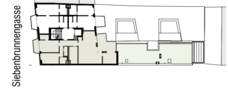
Grundriss 3. Obergeschoss
