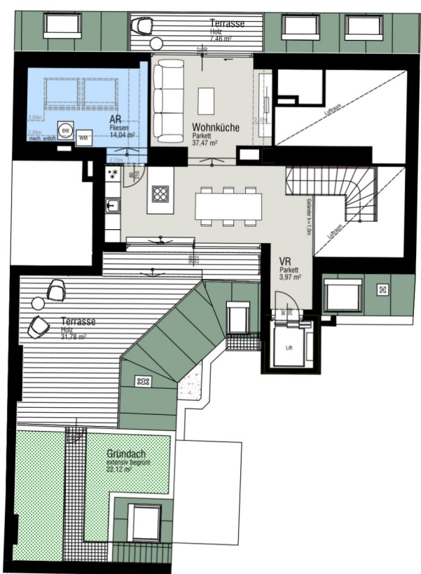
2. DACHGESCHOSS Maßstab 1:200
