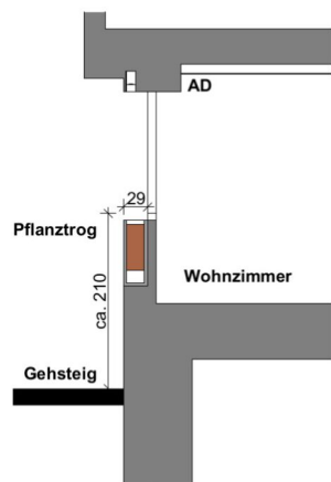
Fassadenschnitt
