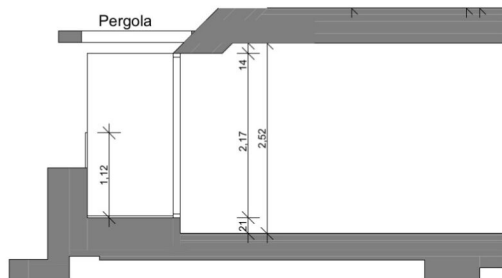
Schnitt 1/73 A
