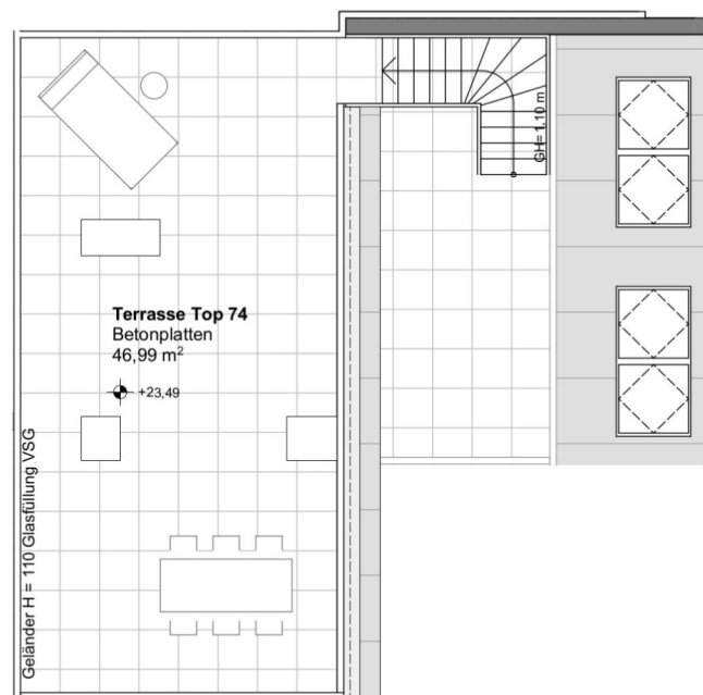
Grundriss Dachterrasse
