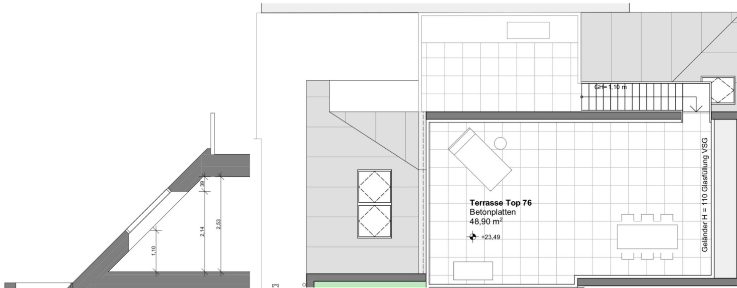
Grundriss Dachterrasse
