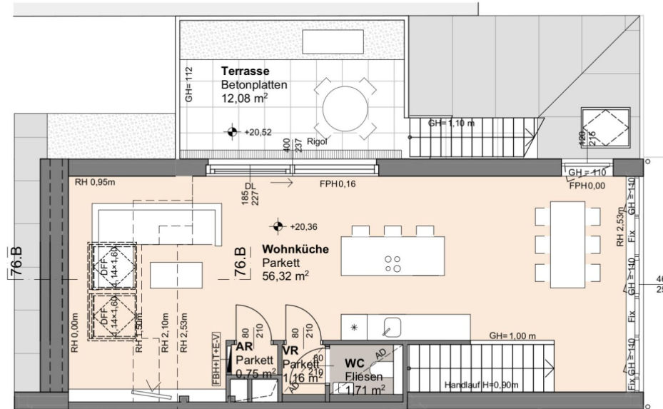
Grundriss 2. Dachgeschoss
