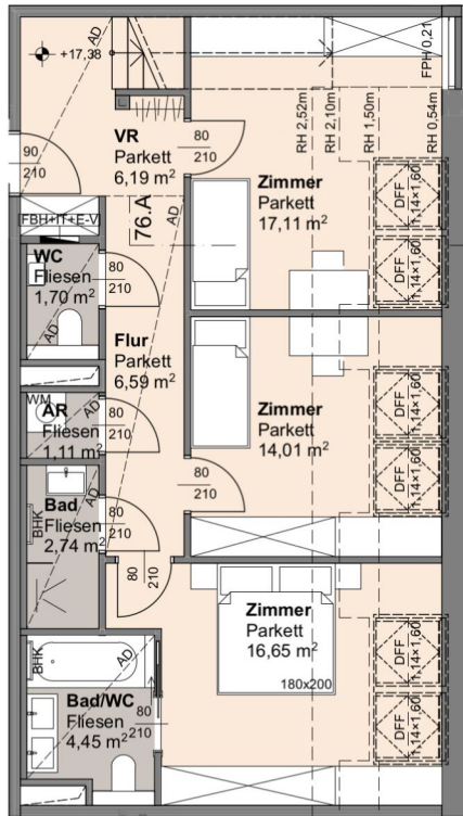
Grundriss 1. Dachgeschoss
