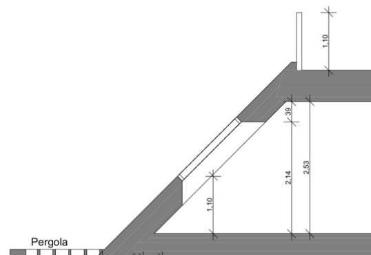
Schnitt 2/71 A
