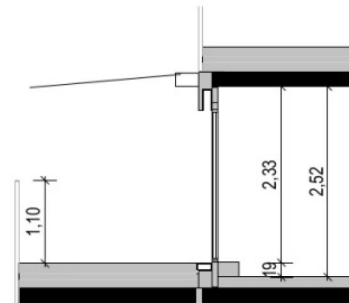
Schnitt 20.A
