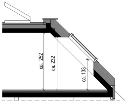
Schnitt 41.A
