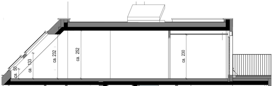
Schnitt 41.B
