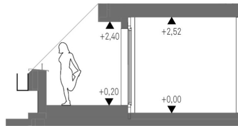
Schnitt 2
