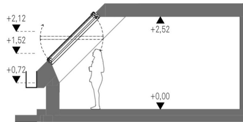
Schnitt 1
