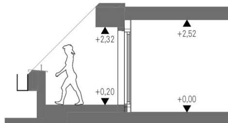
Schnitt 2
