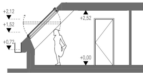
Schnitt 1
