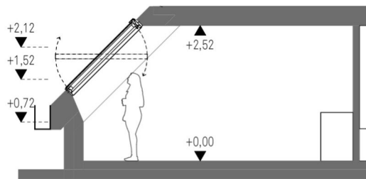
Schnitt 1
