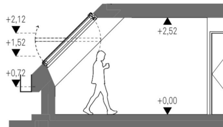
Schnitt 1
