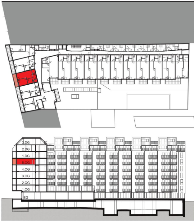
TOP 74 5.OBERGESCHOSS 2 ZIMMER
