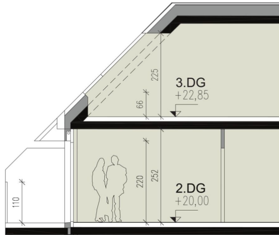
SCHNITT A
