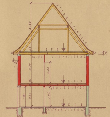
SCHNITT
