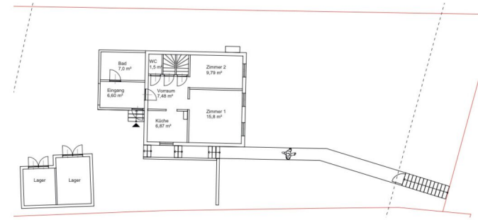
EG
