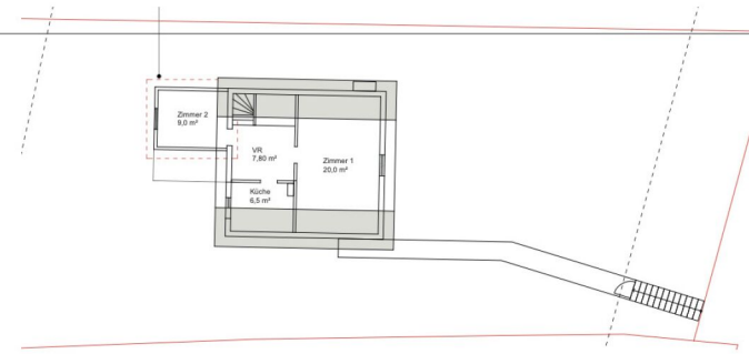
1.OG
