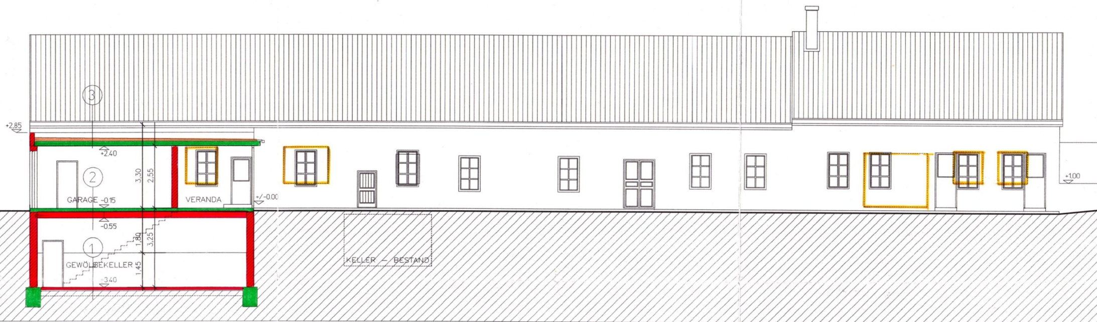
ANSICHT Hof
