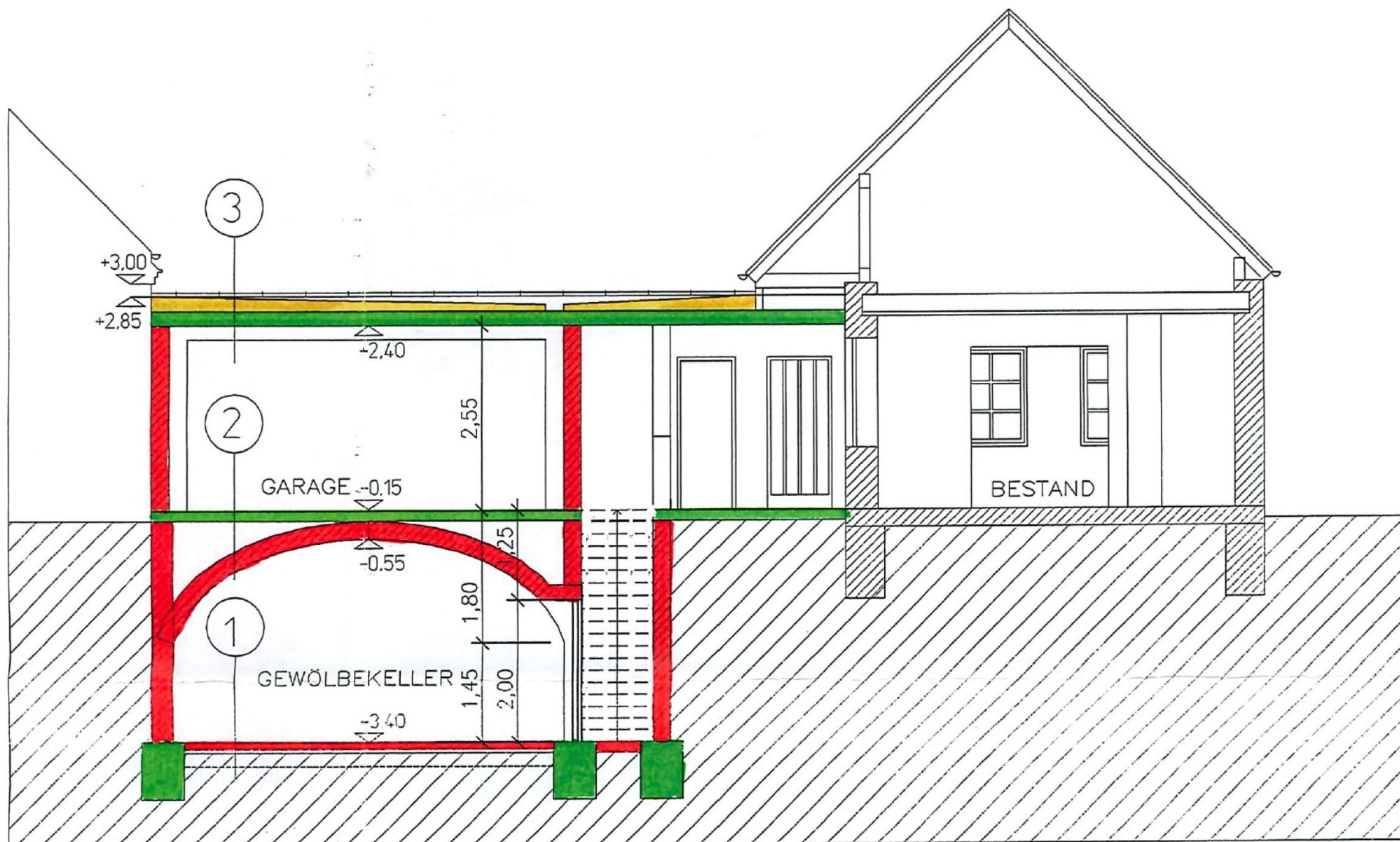
SCHNITT Garage
