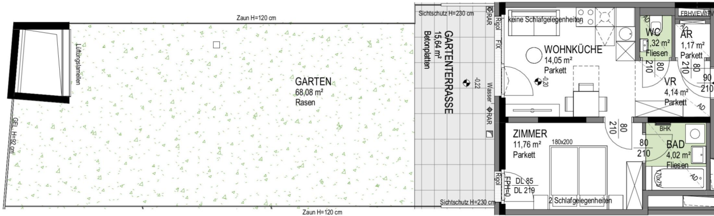
M 1:120
