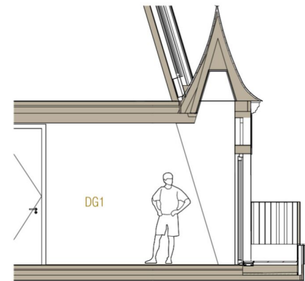
SNITT TOP22
