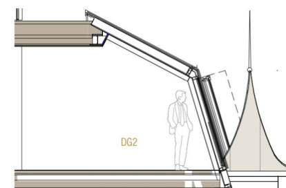
SCHNITT TOP22
