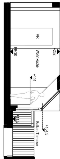
Schnitt S
