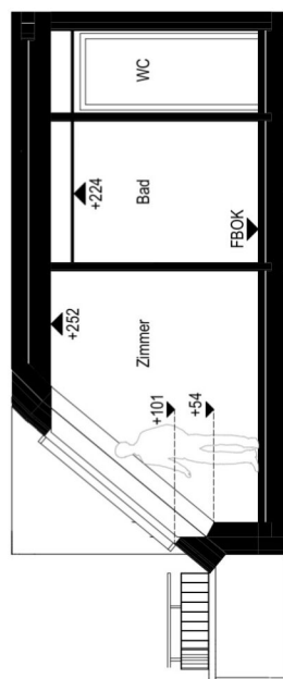
Schnitt S
